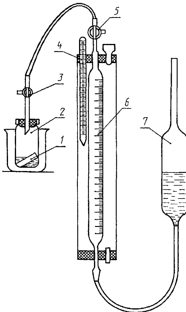
1 - стеклянная пробирка по ГОСТ 25336; 2- сосуд типа СЦ-0,5 по ГОСТ 25336; 3, 5 - краны соединительные по ГОСТ 7995; 4 - термометр по ГОСТ 28498; 6 - бюретка типа 3-2-100-0,2 по ГОСТ 29252-91; 7 - уравнивающая склянка по ГОСТ 25336
