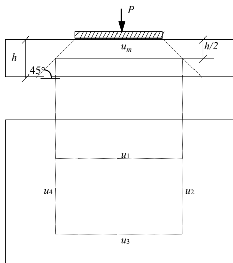
Рис. 3. Схема образования пирамиды при продавливании элемента из арболита
