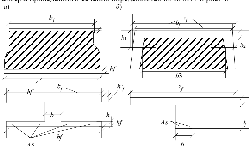
Рис. 4. Схема поперечных сечений составных элементов
